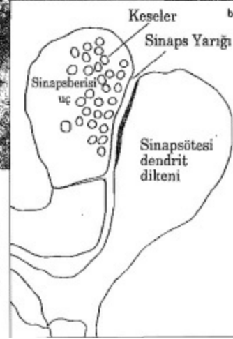
Şekil 34. Elektron mikroskopunda görüldüğü şekliyle diken üzerindeki bir sinapsın incecik bir kesitini görüyorsunuz. Çizim, fotoğraftaki ana öğeleri belirtiyor.
