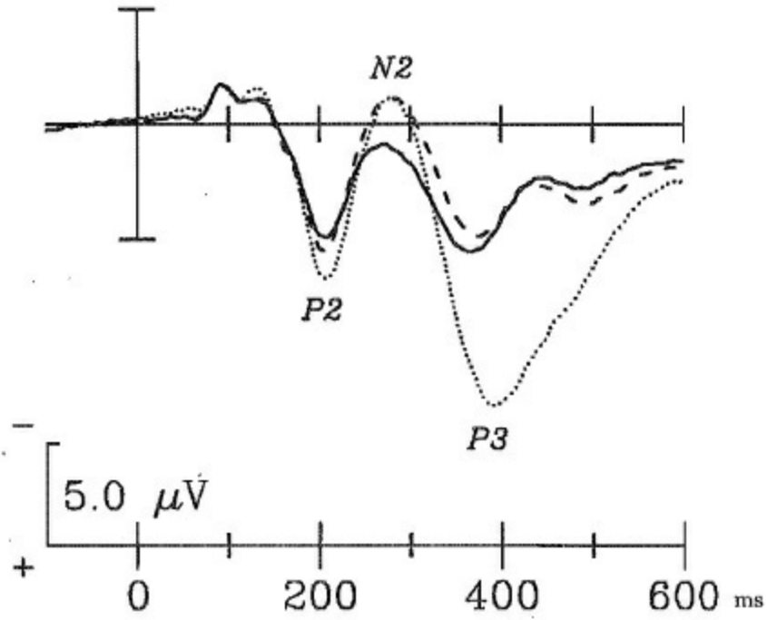
Şekil 35. Ortalama uyarılmış potansiyelin değişik bileşenlerini gösteren eğriler. P300 bileşeni P3 ile gösterilmiştir. Sonuçlar üç olay türüne ait: öne çıkmayan hedef (kesiksiz çizgi), öne çıkmış ama hedef olmayan (kesikli) ve öne çıkmış hedef (noktalı). Sonuncusu için büyük bir P300'un kaydedildiğine dikkat ediniz.
