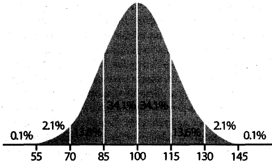
Şekil 1 İstatistik! IQ dağılımı grafiği. Kaynak: Wikipedia
