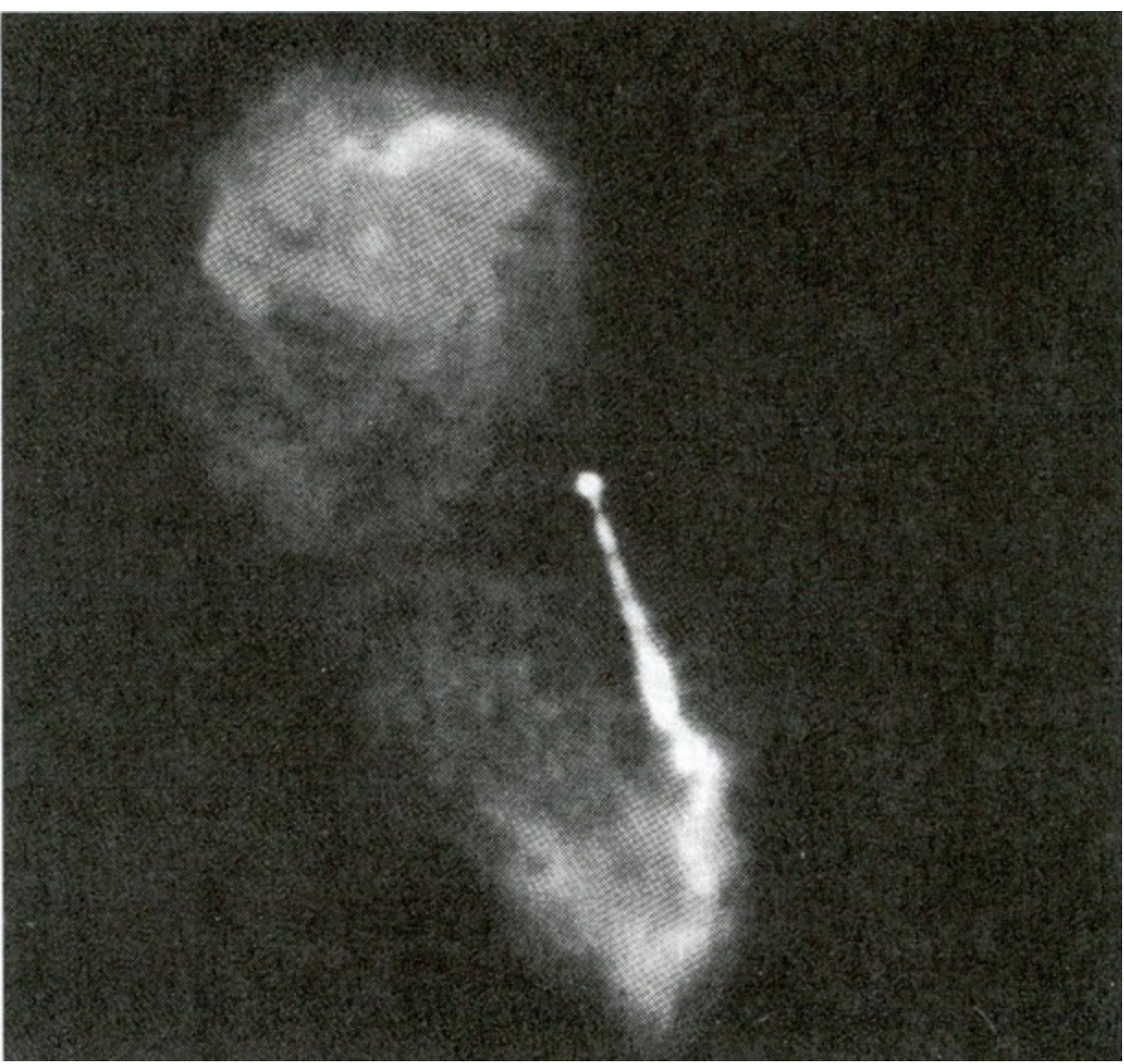
Şekil 15b. M87 galaksisinin radyo dalgalarıyla çekilmiş fotoğrafı. Bir önceki şekilde sönük olarak görünen çizgi, burada açık olarak bir gaz fışkırması biçiminde görülüyor. Fışkırmannın boyu, yaklaşık olarak 5000 ışık yılıdır.
