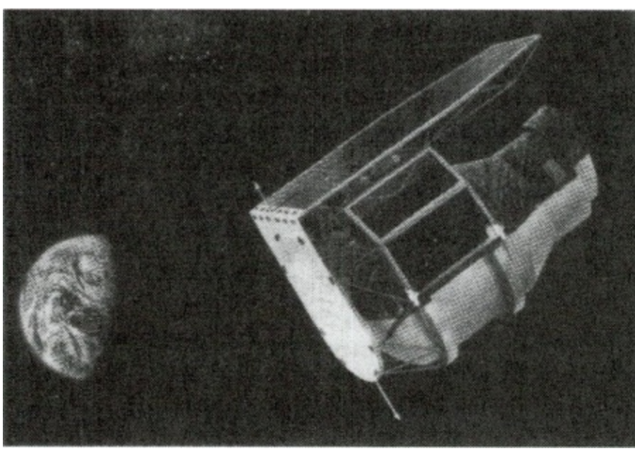
Şekil 5. Dünya çevresindeki yörüngesinde dönecek olan kızılötesi ışınımaya duyarlı Uzay Kızılötesi Teleskopu'nun (SIRTF) hayali görüntüsü.
