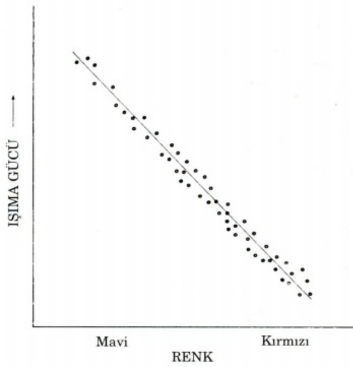
Şekil 8. 'Ana kol' yıldızlarının dağılımı. Her küçük çember, gözlenen bir yıldız temsil ediyor. Yatay eksen, yıldızın gözlenen rengi; dikey eksen ise yıldızın gözlenen ışımaya gücünü gösteriyor. Köşegen doğrultusunda uzanan ve oldukça dar olan kuşağa ana kol adı veriliyor.
