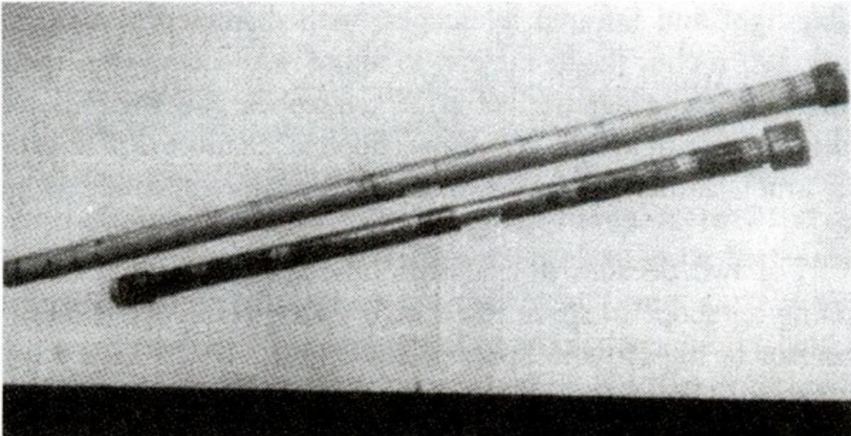
Şekil 14. Galileo'nun, 1610 yılından kalan iki teleskopu. Boyları 1 metre civarında olan bu teleskoplar, Floransa'daki Bilim Tarihi Müzesinde bulunmaktadır.
