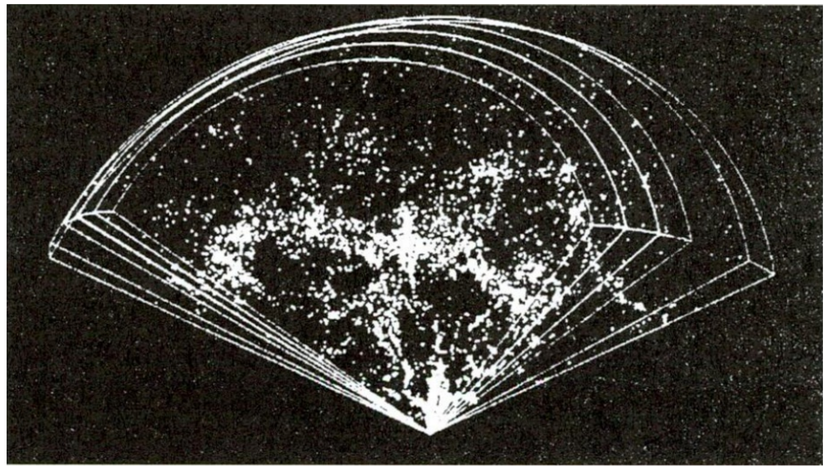
Şekil 16. Astrofizik Merkezinden Margaret Geller ve John Huchra'nın 1989 yılında tamamlanan kırmızıya kayma araştırması. Her nokta bir galaksiyi gösteriyor; burada, birbirine dokunan kama biçimindeki uzay bölgelerinde 3962 galaksi yer alıyor. Yarıçap yönü, homojen bir evrende doğrudan yarıçap yönündeki hız karşılık gelen uzaklaşma hızını gösteriyor. Şekildeki en uzak galaksinin uzaklığı 500 milyon ışık yılıdır. Şeklin ortasında, hemen hemen yatay bir biçimde uzanan galaksi topluluğu, şu ana kadar evrende gözlenen en büyük ve tutarlı galaksi yapılanması olan 'Büyük Duvar'dır.
