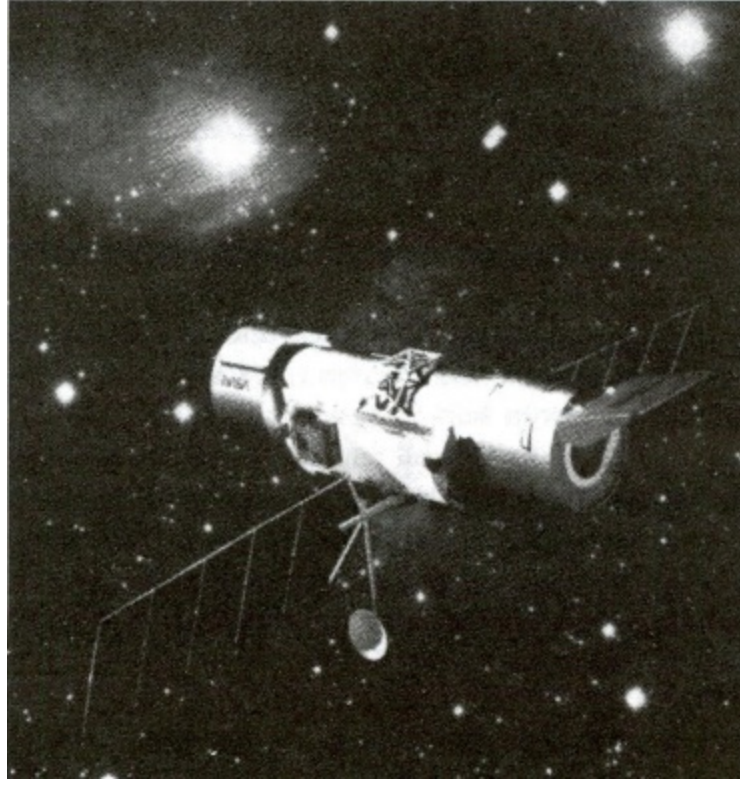
Şekil 10. Dünya çevresindeki yörüngesinde dönecek olan, X-ışınlarına duyarlı İleri X-Işını Astrofizik Uydusunun (AXAF) hayali görüntüsü
