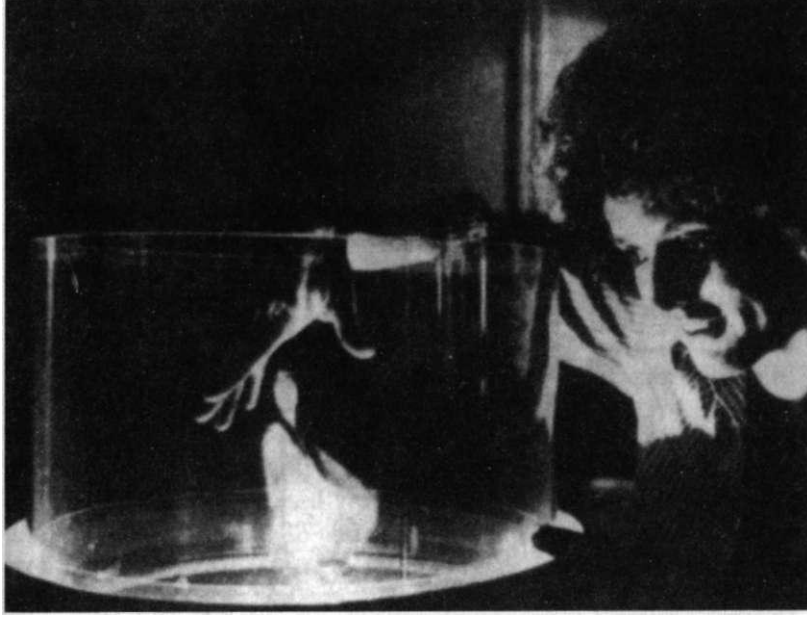
Resim 3: Bir hologramın üç boyutlu imgesi bazen insanı ürkütecek denli inandırıcıdır, onun çevresinde dolaşabilir ve ona farklı açılardan bakabilirsiniz. Ama elinizi uzatıp dokunmaya kalkışacak olursanız parmaklarınız içinden geçer. ("Çıplak Celeste" 1978'de Peter Claudius tarafından oluşturulmuş bir holografik stereogram. Brad Cantos tarafından çekilmiş olan fotoğraf Holografi Müzesinin koleksiyonunda bulunmaktadır.)
