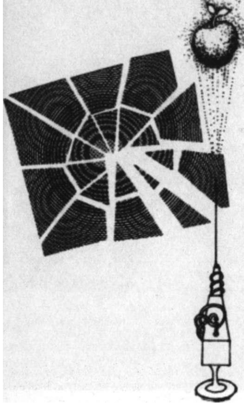
Resim 4: Normal fotoğrafların tersine holografik filmin her bir parçası, filmin tümüne kayıtlı bulunan bilgileri kapsar. Böylece bir holografik plâka, parçalara ayrılmış bile olsa, her parça tüm bir imgeyi oluşturmakta yine de kullanılabilir.
