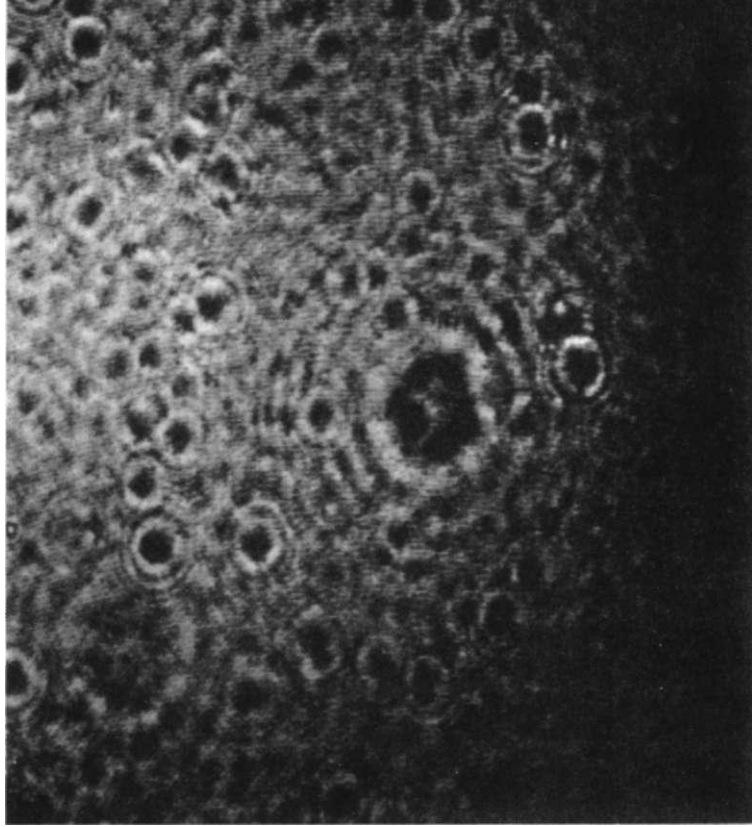
Resim 2: Üzerine bir imge şifrelenmiş bir holografik film parçası. Çıplak gözle bakıldığında film üzerindeki imgenin, fotoğrafı çekilen nesneyle hiçbir ilgisi yoktur, girişim deseni diye adlandırılan dağınık dalgacıklardan oluşmuş gibi görünmektedir. Ancak film başka bir lazerle aydınlatıldığında orijinal nesnenin üç boyutlu bir imgesi ortaya çıkar.
