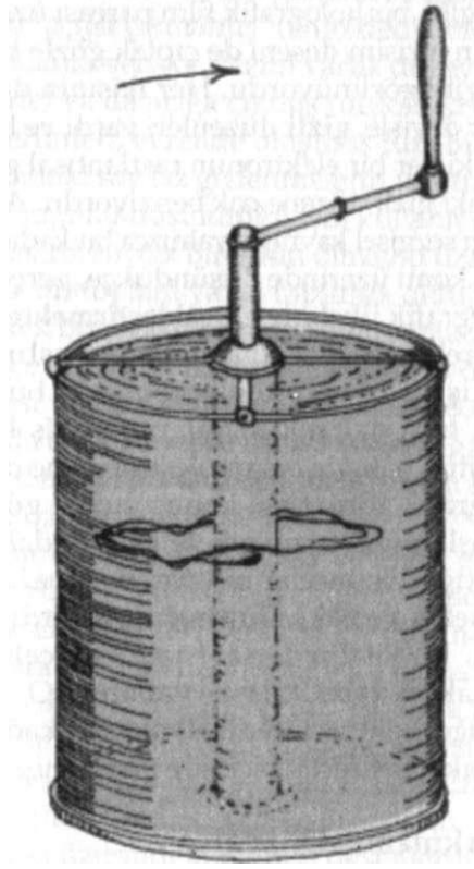
Resim 9: Gliserin dolu bir kavanozun içinde bir mürekkep damlası yerleştirildikten sonra kavanozun içindeki silindiri döndürülecek olursa, bu damla yayılır ve gözden kaybolur. Ama silindiri ters yönden döndürdüğümüzde damla yeniden biraraya gelir. Bohm, bu fenomeni düzenin nasıl ortaya çıktığını (belirginleştiğini) ve nasıl gözden saklandığını (gizlendiğini) gösterebilmek için bir örnek olarak kullanmıştır.
