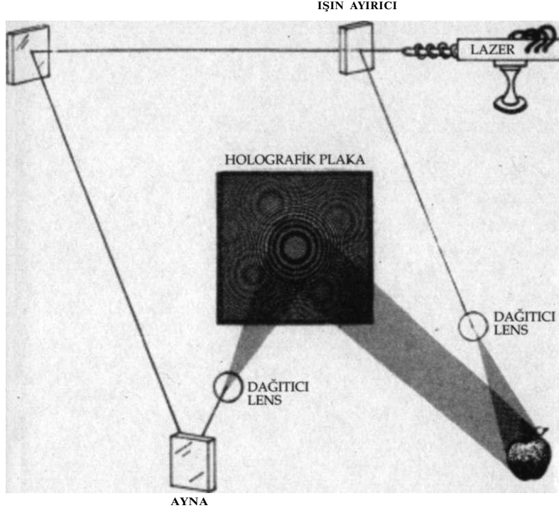
Resim 1: Bir hologram tek bir lazer ışını iki ayrı ışına ayırılarak oluşturulur. İlk ışın fotoğrafı çekilecek nesneden (bu örnekte bir elmadır) sektirilir. Sonra ikinci ışın ilkinin yansıyan ışığıyla çarpıştırılır ve ortaya çıkan girişim deseni filme kaydedilir.
