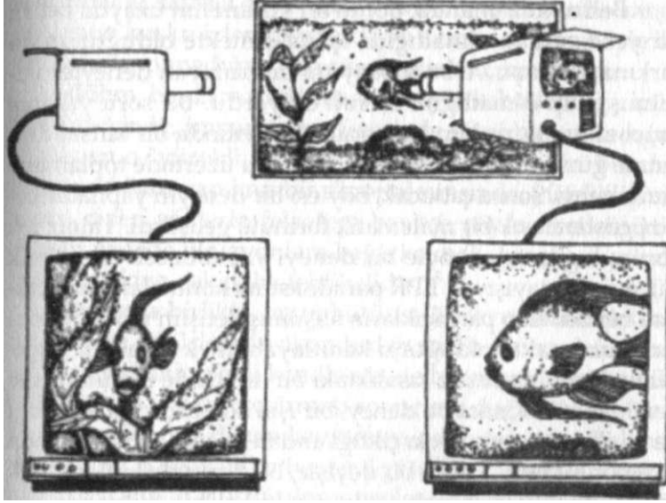
Resim 8: Bohm, atomal parçacıklarının birbirleriyle, iki televizyon monitöründen yansıyan bir balığın imgeleri kadar ilişkili olduğuna inanıyor. Birbirlerinden ayrıymış gibi görünen elektronlara benzer parçacıklar, daha derin bir gerçeklik düzeyinde -akvaryumun içine benzer bir düzeyde- yalnızca daha derin bir kozmik birliğin farklı görünümleriydi.
